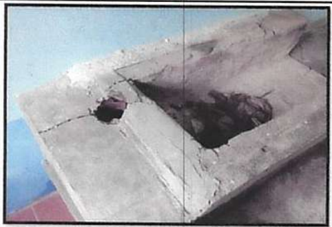
Foto 9: Reconstrucción de estufa con plancha y chimenea
